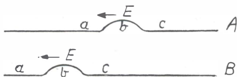
Fig. 1. Dos etapas del traslado de una onda corriente transversal, A y B son dos etapas del movimiento. "a" es la fibra no disturbada, "b" es la onda, "c" es la fibra no disturbada, E es la energía de la onda que se mueve con la misma. La flecha demuestra la dirección de propagación de la onda corriente transversal.
